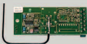
Steckplatz für optionalen ELKA-Funkempfänger, 434MHz, Kanal 1 für Vollöffnung Kanal 2 für Teilöffnung
